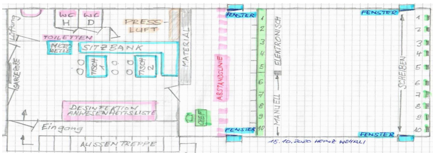
Abbildung: angenäherte Grobskizze P10M-, bzw. G10M -Anlage Pappelweg
