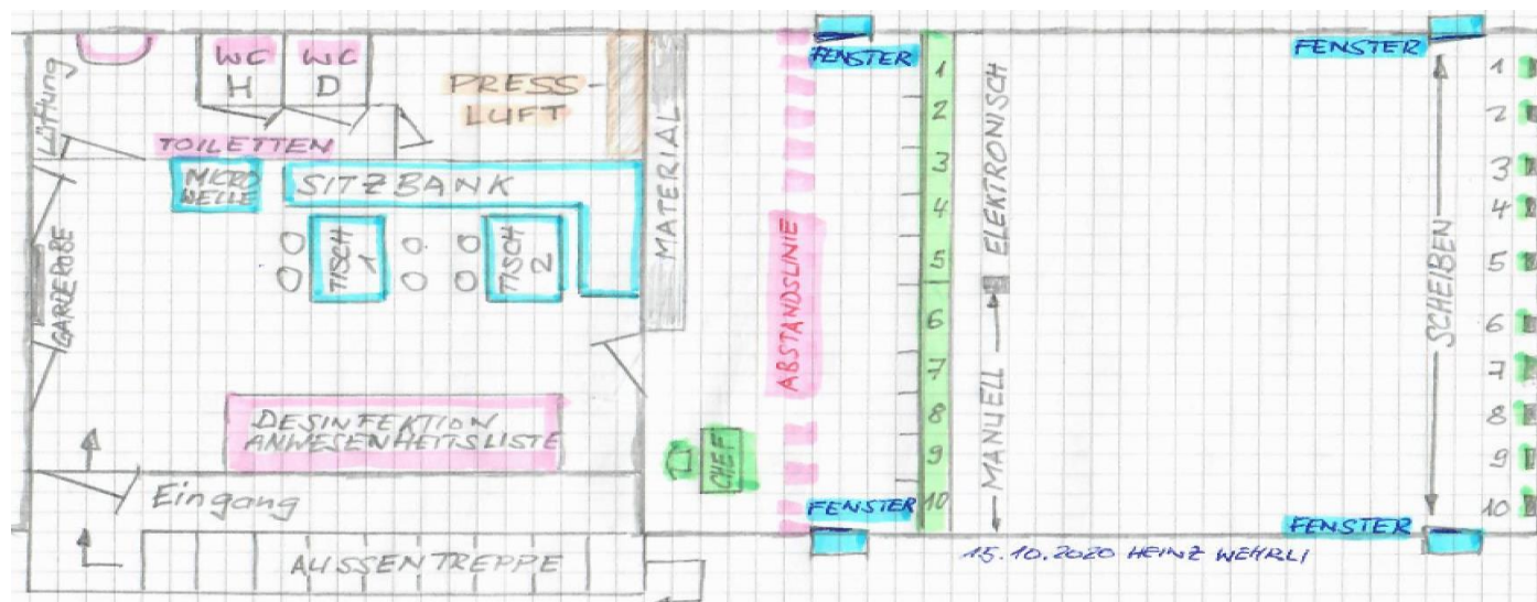
Abbildung: angenäherte Grobskizze P10M-, bzw. G10M -Anlage Pappelweg
